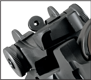
ALÇA DE MIRA COM ABERTURA TIPO MILITAR COM .069" - AJUSTE LATERAL E ALTURA EM MOA
