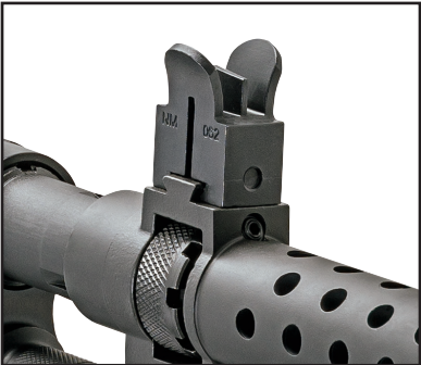
MASSA DE MIRA NATIONAL MATCH EM LÂMINA .062”
