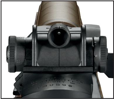
ALÇA DE MIRA DE COMPETIÇÃO SEM PROTEÇÃO SUPERIOR COM ABERTURA .0595” COM AJUSTES LATERAIS DE ½ MOA & ½ MOA NA ALTURA
