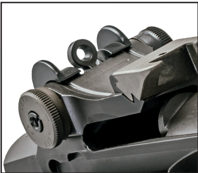
MASSA DE MIRA COM ABERTURA TIPO MILITAR COM .135" - AJUSTE LATERAL E ALTURA EM MOA
