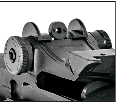
ALÇA DE MIRA DE COMPETIÇÃO SEM PROTEÇÃO SUPERIOR COM ABERTURA .0520" COM AJUSTES LATERAIS DE 1/2 MOA & 1/2 MOA NA ALTURA
