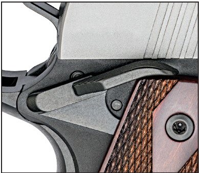
TRAVA DE SEGURANÇA AMBIDESTRA
