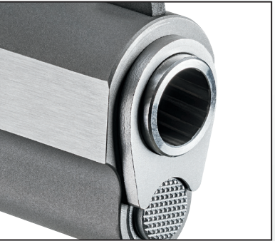
CANO E BUCHA DO CANO EM AÇO INOXIDÁVEL
